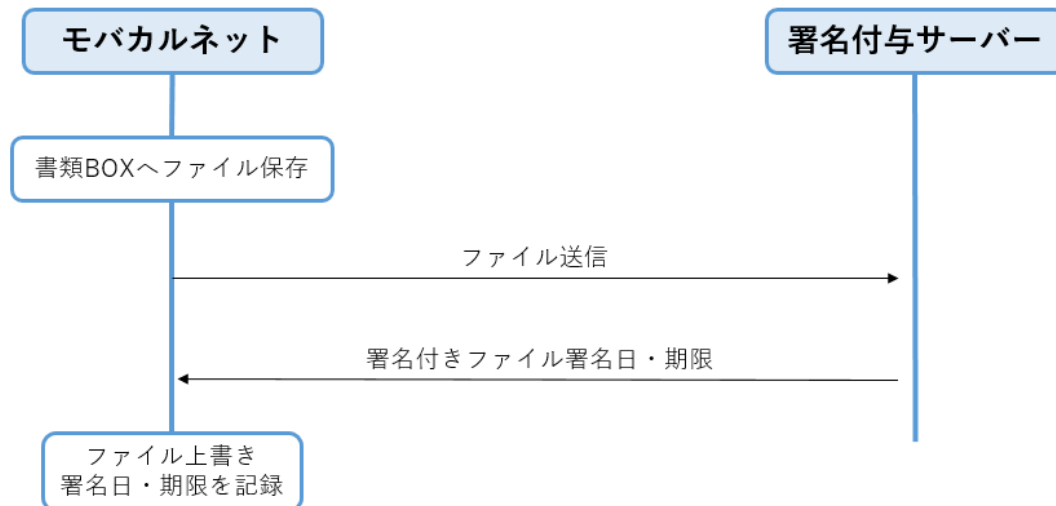
図 1-1 システム構成図
